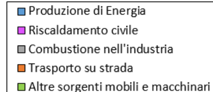
Emissioni di NO x per tipologia di combustibile
