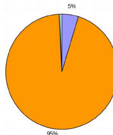
Emissioni di NO x per tipologia di combustibile
