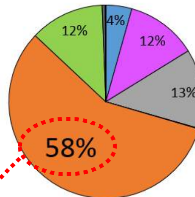
Emissioni di NO x per macrosettore
