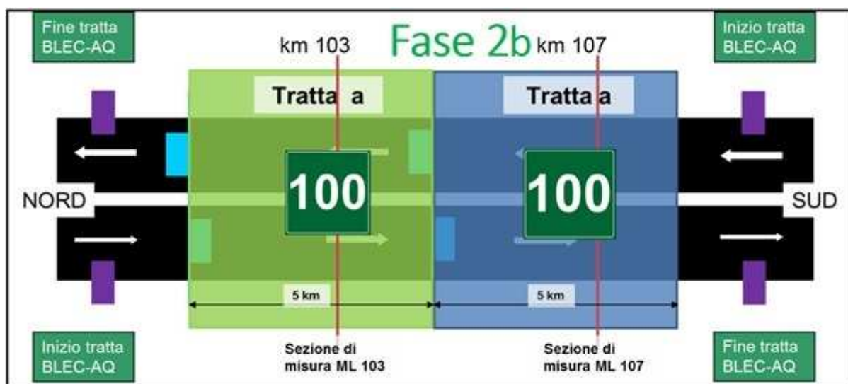
Figura 3: Allestimento del sito di test BLEC-AQ per la seconda fase di test con i limiti dinamici di velocità per fini ambientali utilizzato da dicembre 2018 fino a settembre 2019.
