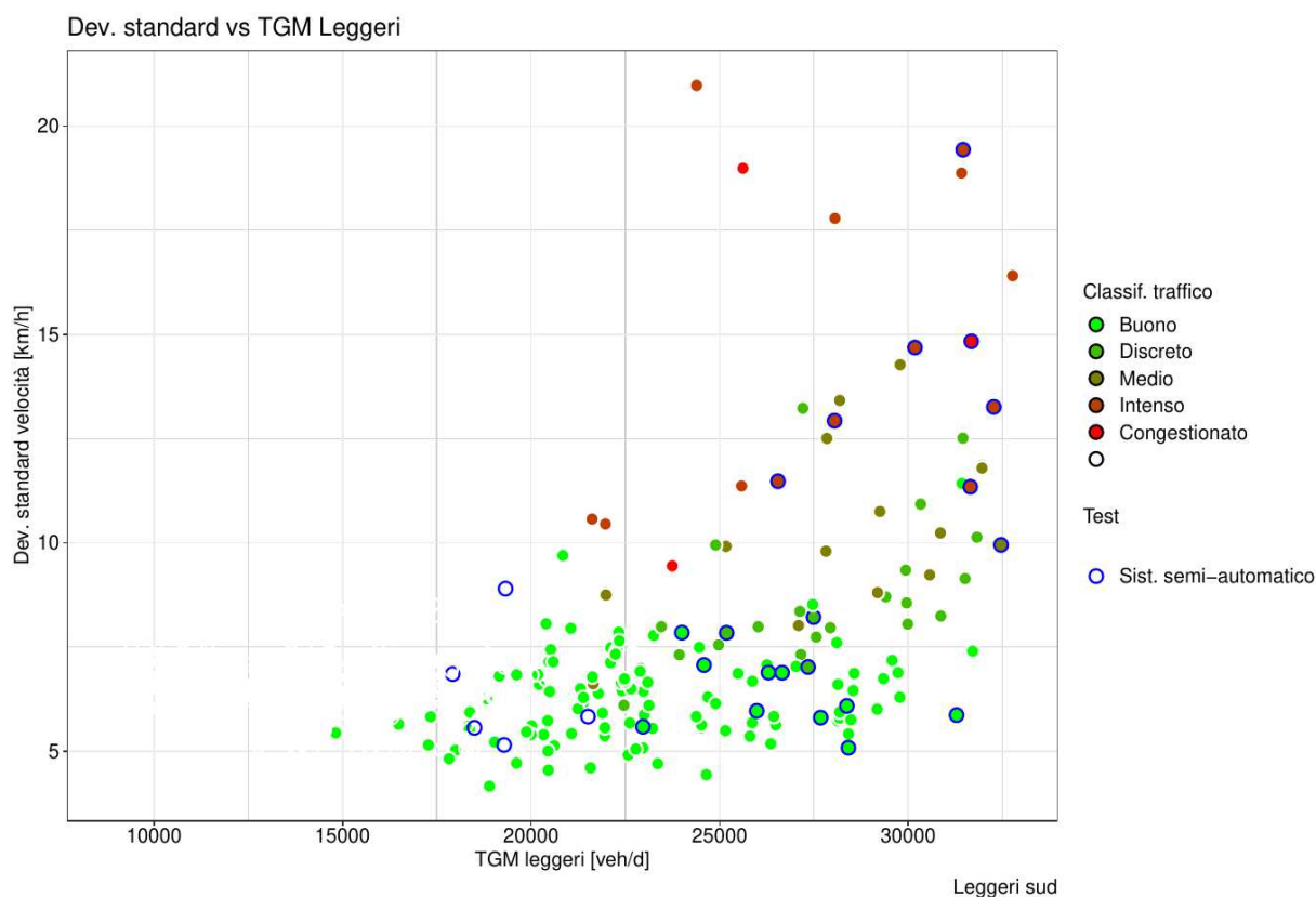
Figura 28: Classificazione del traffico, deviazione standard della velocità, numero di transiti di veicoli leggeri misurati presso la spira al km 164 dal 18/04/2018 e presenza del sistema semi-automatico- valori medi giornalieri.
