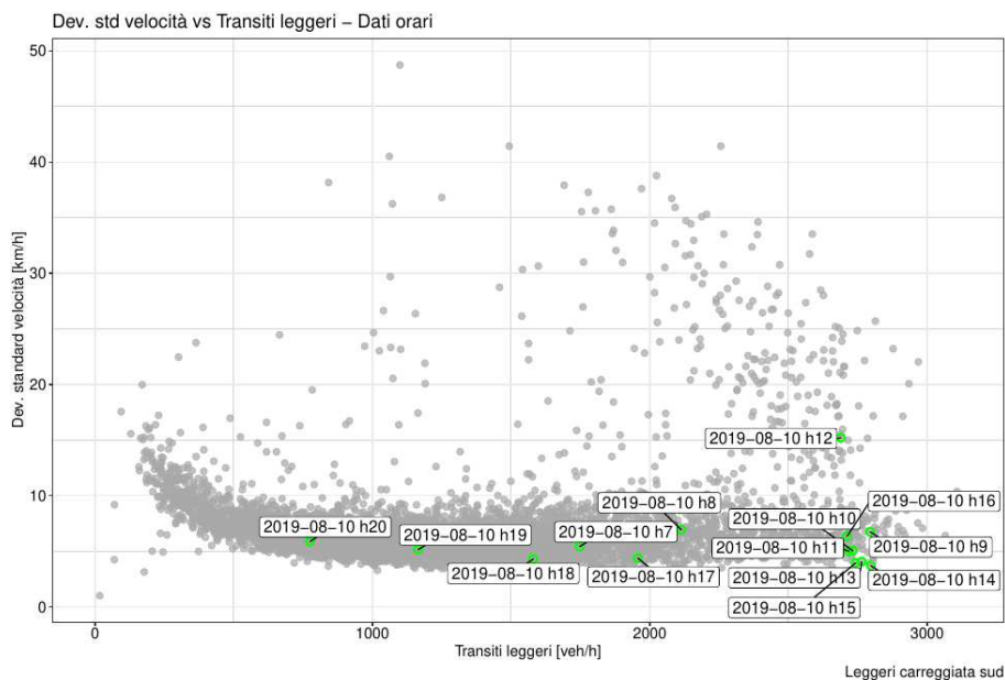
Figura 23: Grafico dei dati orari di deviazione standard della velocità e del numero di transiti di veicoli leggeri
