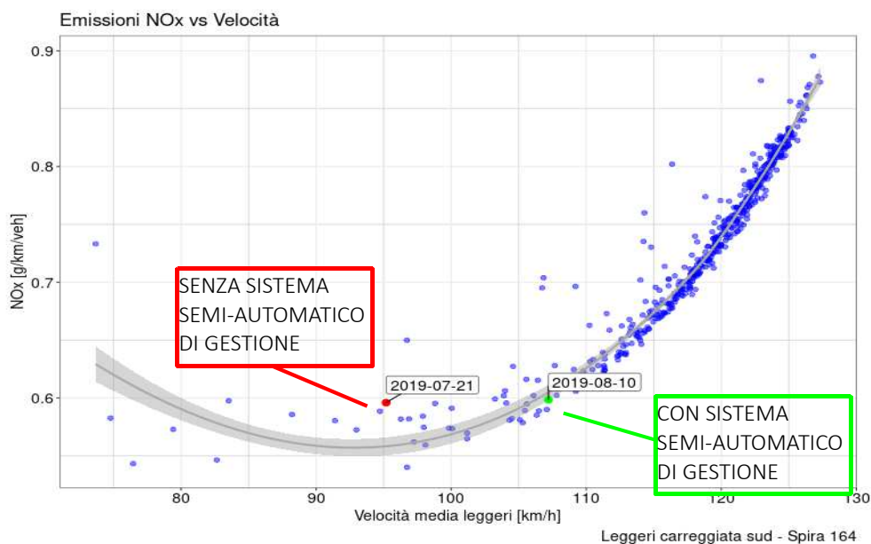
Figura 31: Emissioni di ossidi di azoto durante ciascuna giornata di test per veicolo leggero per chilometro di tratta percorsa.
