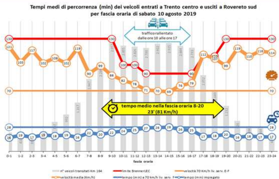
Figura 17: Riassunto delle principali variabili trasportistiche rilevate il 10 agosto 2019.
