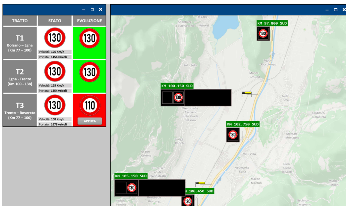
Figura 13: Interfaccia del sistema di gestione semi-automatica dei limiti di velocità.
