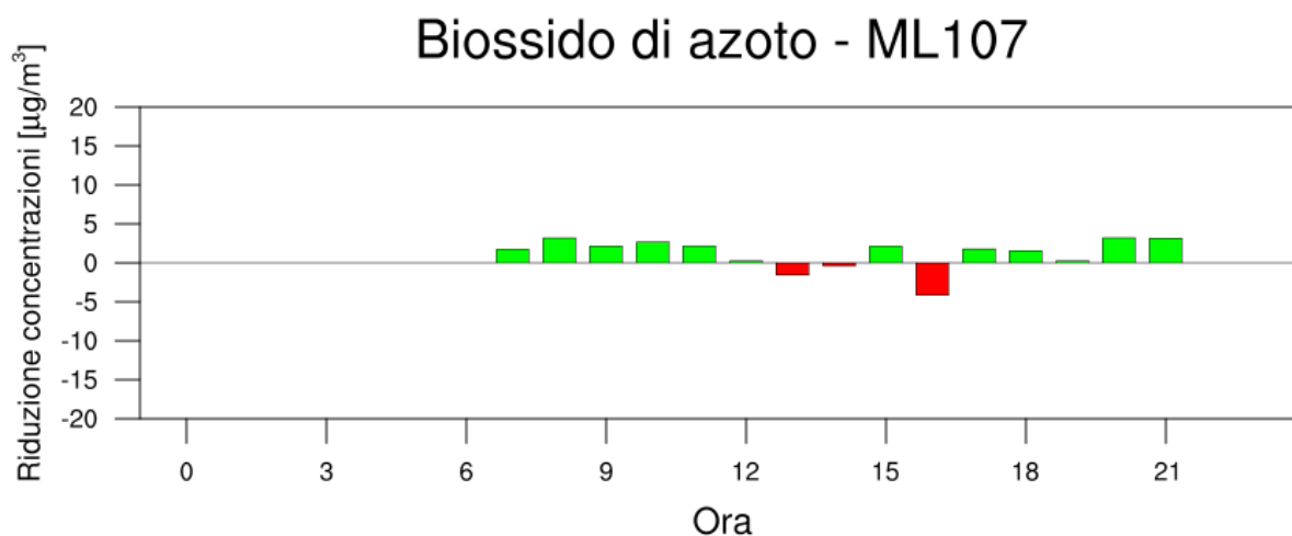
Figura 9: Benefici ambientali ottenuti durante i test di fase 2 alla stazione ML107 per quanto riguarda il biossido di azoto.
