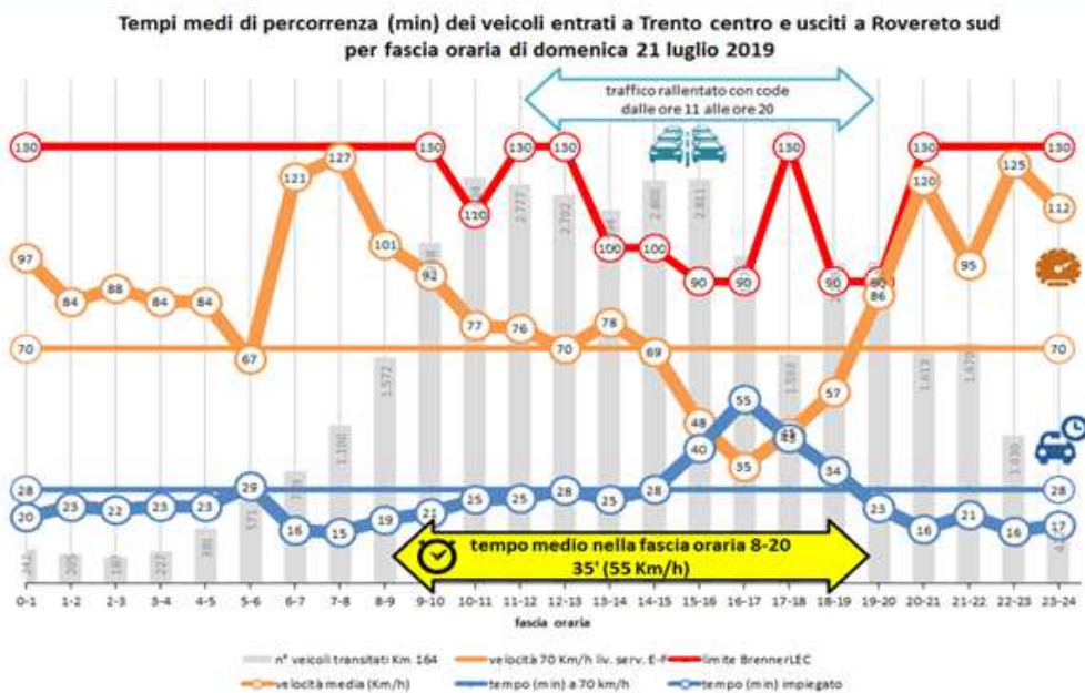
Figura 16: Riassunto delle principali variabili trasportistiche rilevate il 21 luglio 2019.
