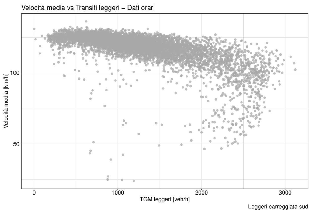
Figura 18: Grafico dei dati orari di velocità media e del numero di transiti di veicoli leggeri misurati presso la spira al km 164 dal 18/04/2018.
