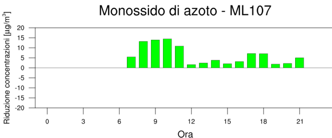
Figura 7: Benefici ambientali ottenuti durante i test di fase 2 alla stazione ML107 per quanto riguarda il monossido di azoto.
