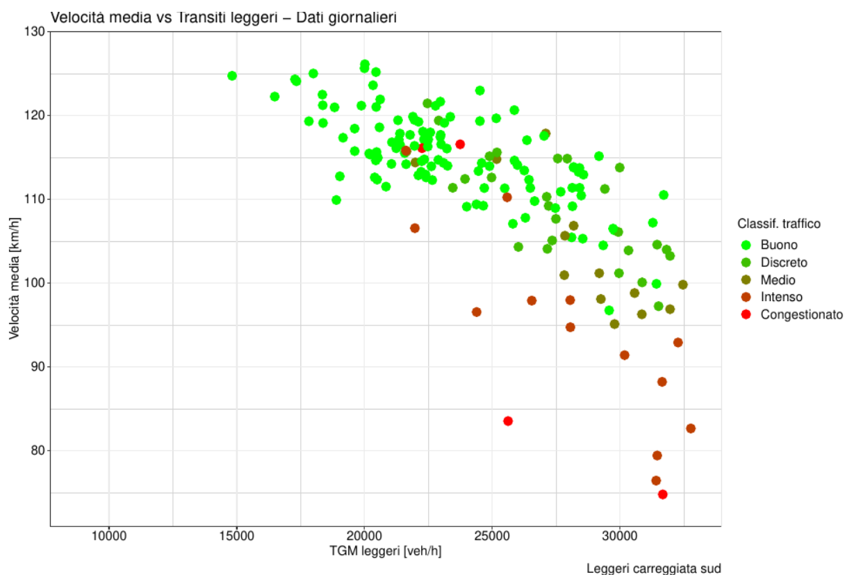
Figura 26: Classificazione del traffico, velocità media e numero di transiti di veicoli leggeri misurati presso la spirale al km 164 dal 18/04/2018 - valori medi giornalieri.
