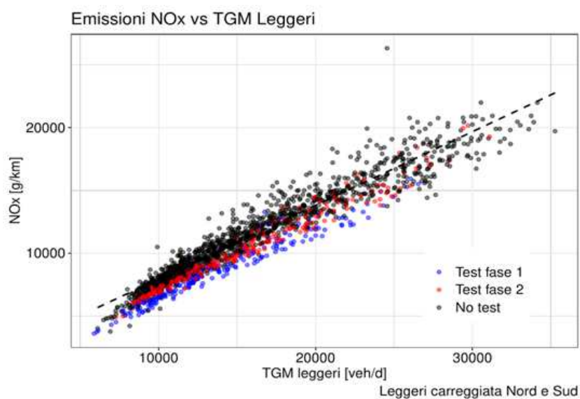
Figura 10: Emissioni di ossidi di azoto [g/km] in funzione del numero totale giornaliero di veicoli leggeri durante i test di fase 1 (punti blu), i test di fase 2 (punti rossi) e le giornate senza test (punti neri).
