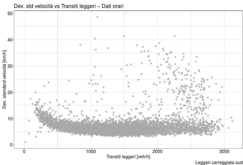
Figura 19: Grafico dei dati orari di deviazione standard della velocità e del numero di transiti di veicoli leggeri misurati presso la spira al km 164 dal 18/04/2018.
