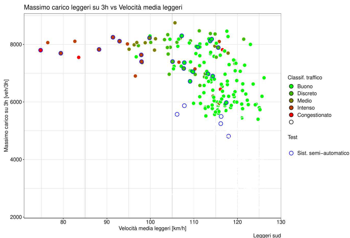
Figura 29: Classificazione del traffico, massimo carico di veicoli leggeri su tre ore e numero totale di transiti di veicoli leggeri misurati presso la spira al km 164 dal 18/04/2018 e presenza del sistema semi-automatico- valori giornalieri.
