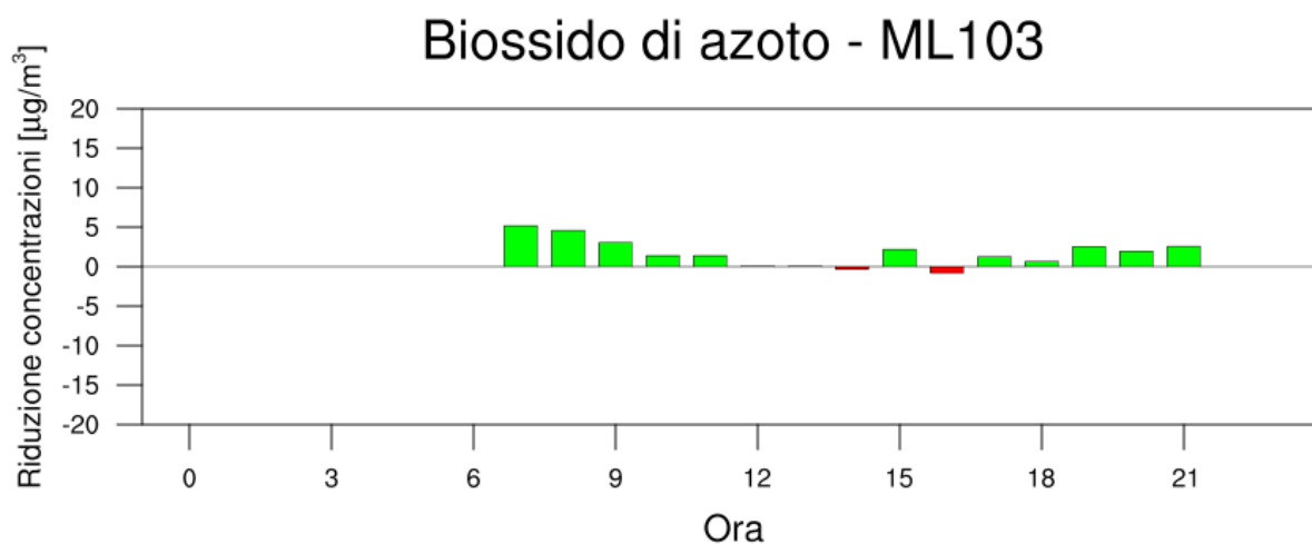
Figura 8: Benefici ambientali ottenuti durante i test di fase 2 alla stazione ML103 per quanto riguarda il biossido di azoto.
