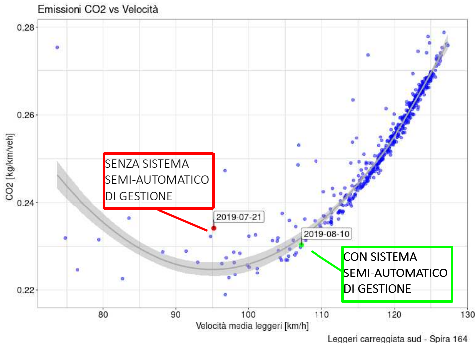
Figura 30: Emissioni di biossido di carbonio durante ciascuna giornata di test per veicolo leggero per chilometro di tratta percorsa.
