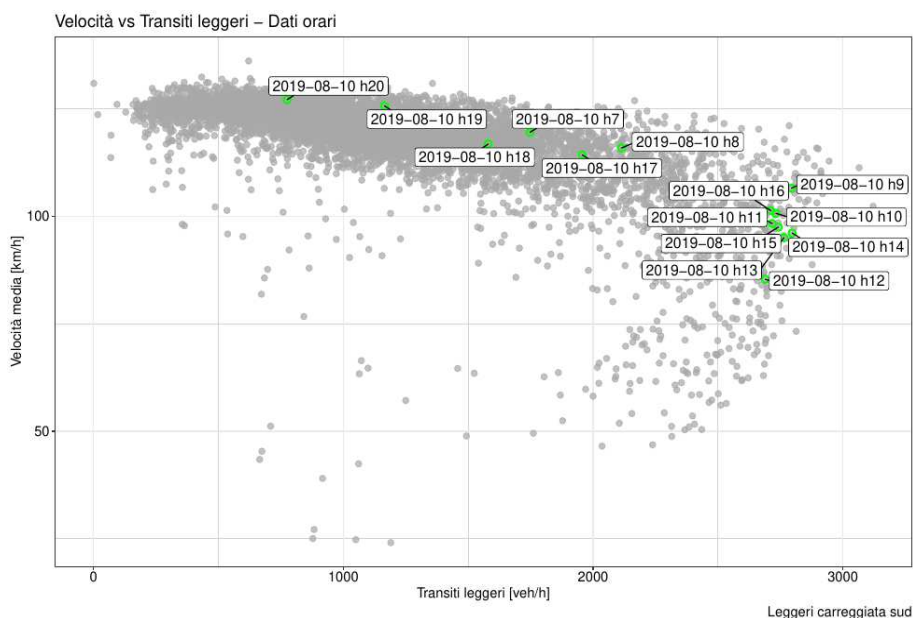
Figura 22: Grafico dei dati orari di velocità media e del numero di transiti di veicoli leggeri misurati presso la spira al km 164 dal 18/04/2018 in cui sono evidenziate le ore relative alla giornata del 10/08/2019.
