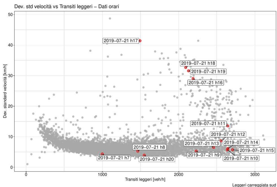
Figura 21: Grafico dei dati orari di deviazione standard della velocità e del numero di transiti di veicoli leggeri
