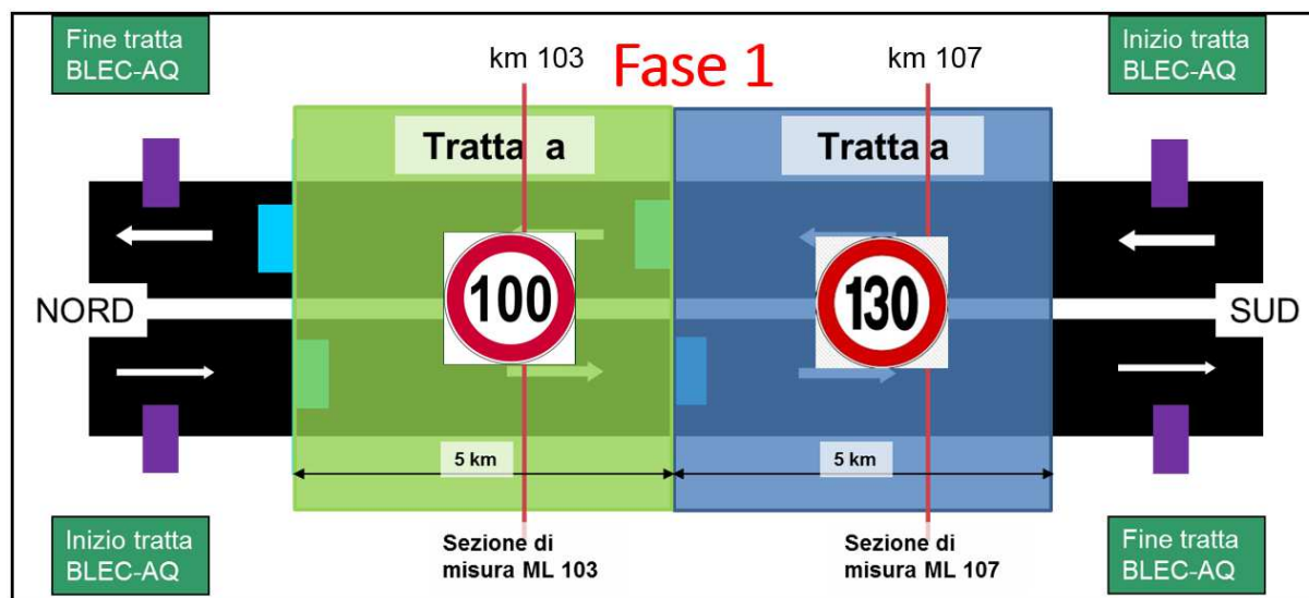
Figura 1: Allestimento del sito di test BLEC-AQ per la prima fase di test con i limiti dinamici di velocità per fini ambientali.
