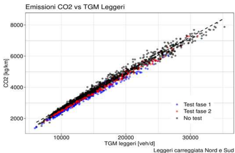
Figura 11: Emissioni di biossido di carbonio [g/km] in funzione del numero totale giornaliero di veicoli leggeri durante i test di fase 1 (punti blu), i test di fase 2 (punti rossi) e le giornate senza test (punti neri).
