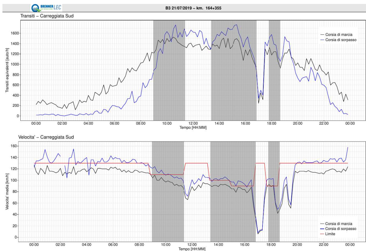
Figura 24: Andamento temporale dei transiti di veicoli leggeri e delle velocità medie presso la spira al km 164 nella giornata del 21/07/2019.
