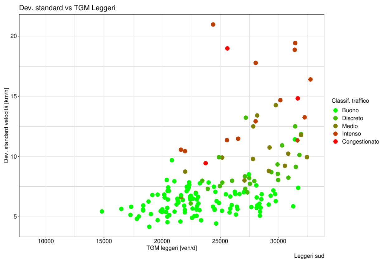
Figura 27: Classificazione del traffico, deviazione standard della velocità e numero di transiti di veicoli leggeri misurati presso la spira al km 164 dal 18/04/2018- valori medi giornalieri.
